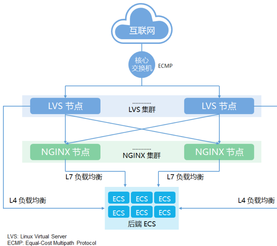
图 6-2 华为云 ELB 组网图
